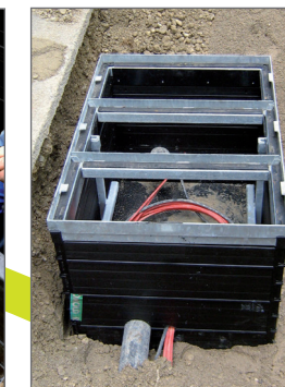
Prostopadłe przyłączenie rur
