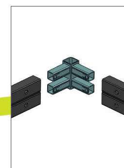
Podzielna w pionie, profil z narożnym łącznikiem, otwór drenażowy w płycie dolnej
