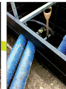
Możliwość wprowadzania rur pod kątem
