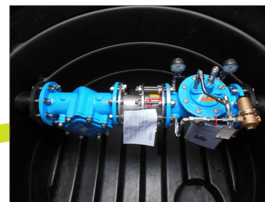
Studnia z zaworem redukcji ciśnienia
