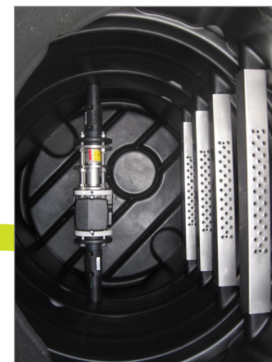
Studnia wodomierzowa ze zintegrowanym miernikiem przepływu MID
